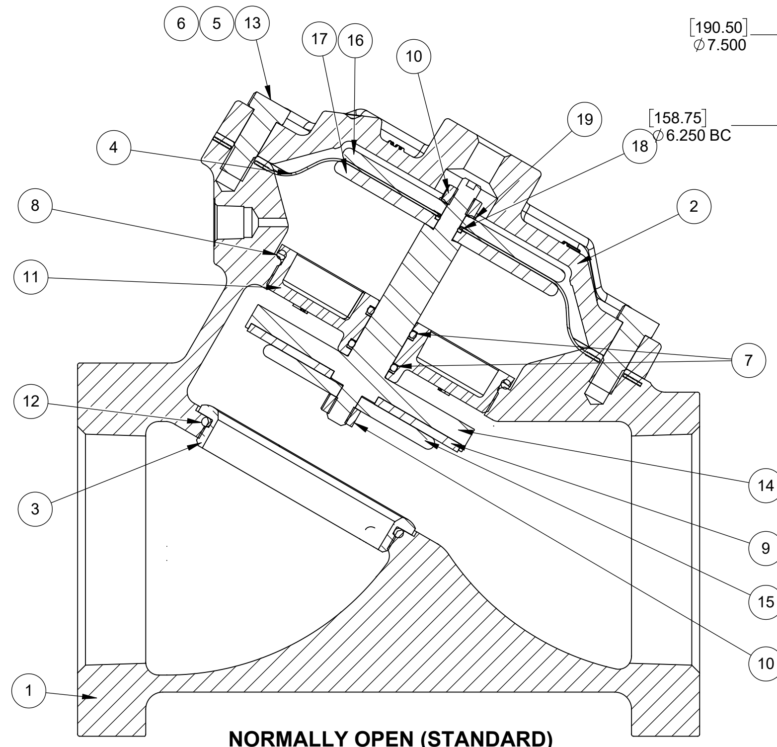
METRIC FLANGE PER BS4504. DIN 10 & ISO R 2084
